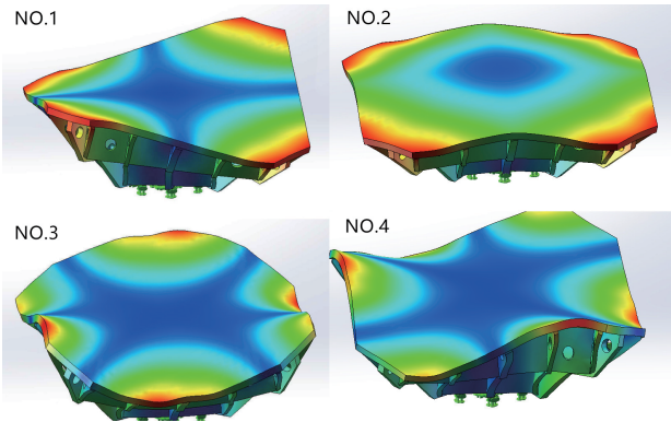
— 模态仿真图 —
