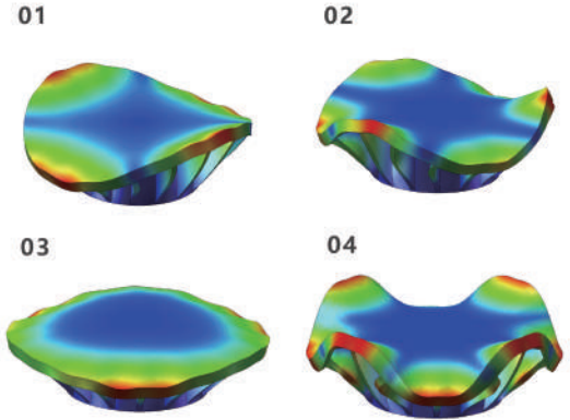
- 模态仿真图 -
