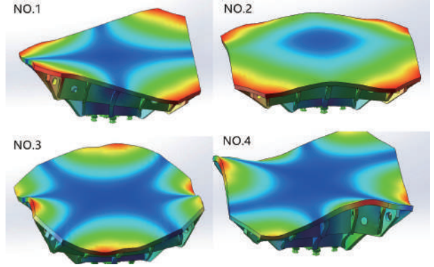
- 模态仿真图 -
